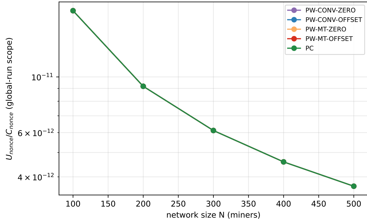
Unique nonce-value fraction: 2^{32} values / total evaluations
