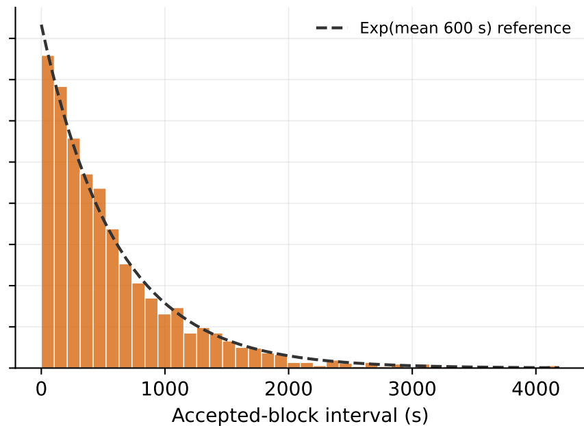
X-PC (PoCol)
