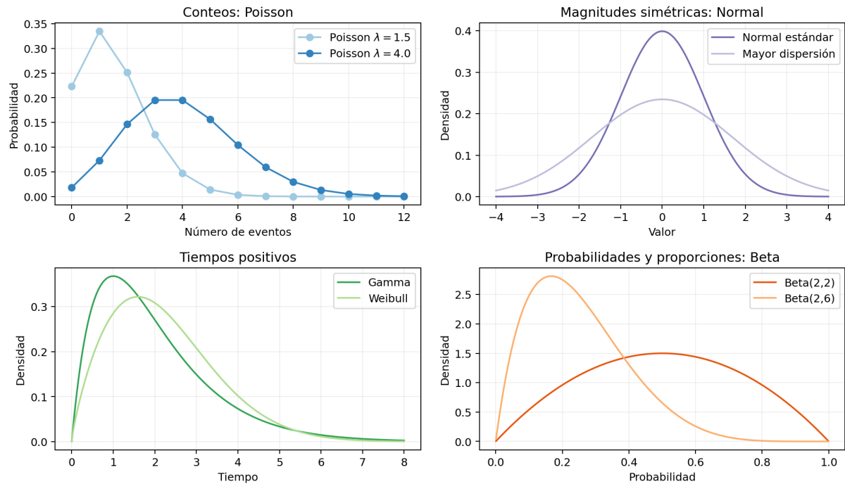
Figura 10: Ejemplos de distribuciones probabilísticas
