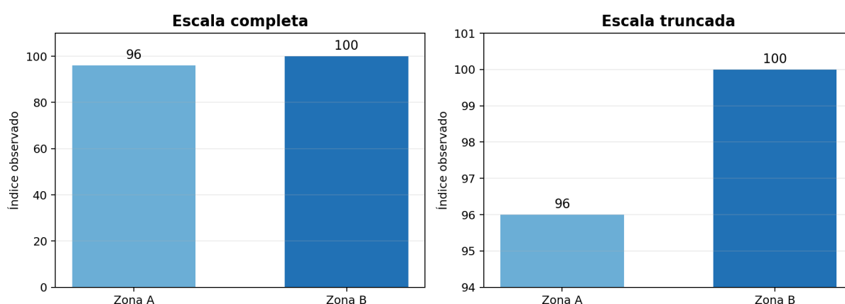
Figura 9: Efecto de una escala truncada
