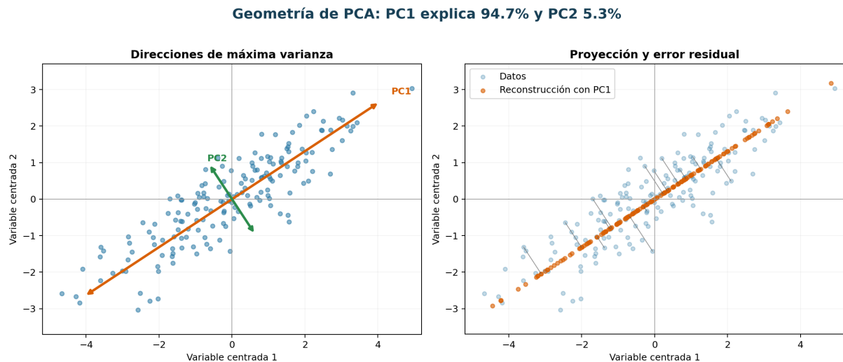
Figura 13: Geometría de PCA: ejes principales, proyección y reconstrucción
