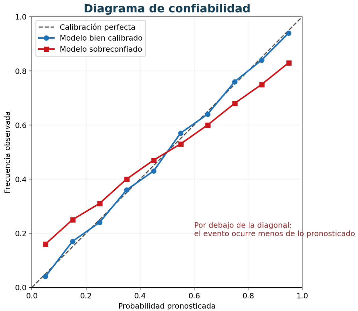
Figura 12: Ejemplo de calibración probabilística
