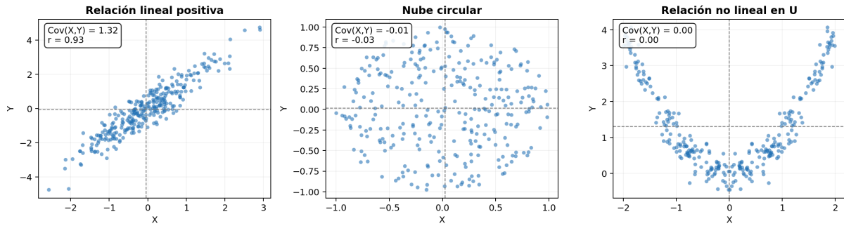
Figura 5: Interpretación geométrica de la covarianza
