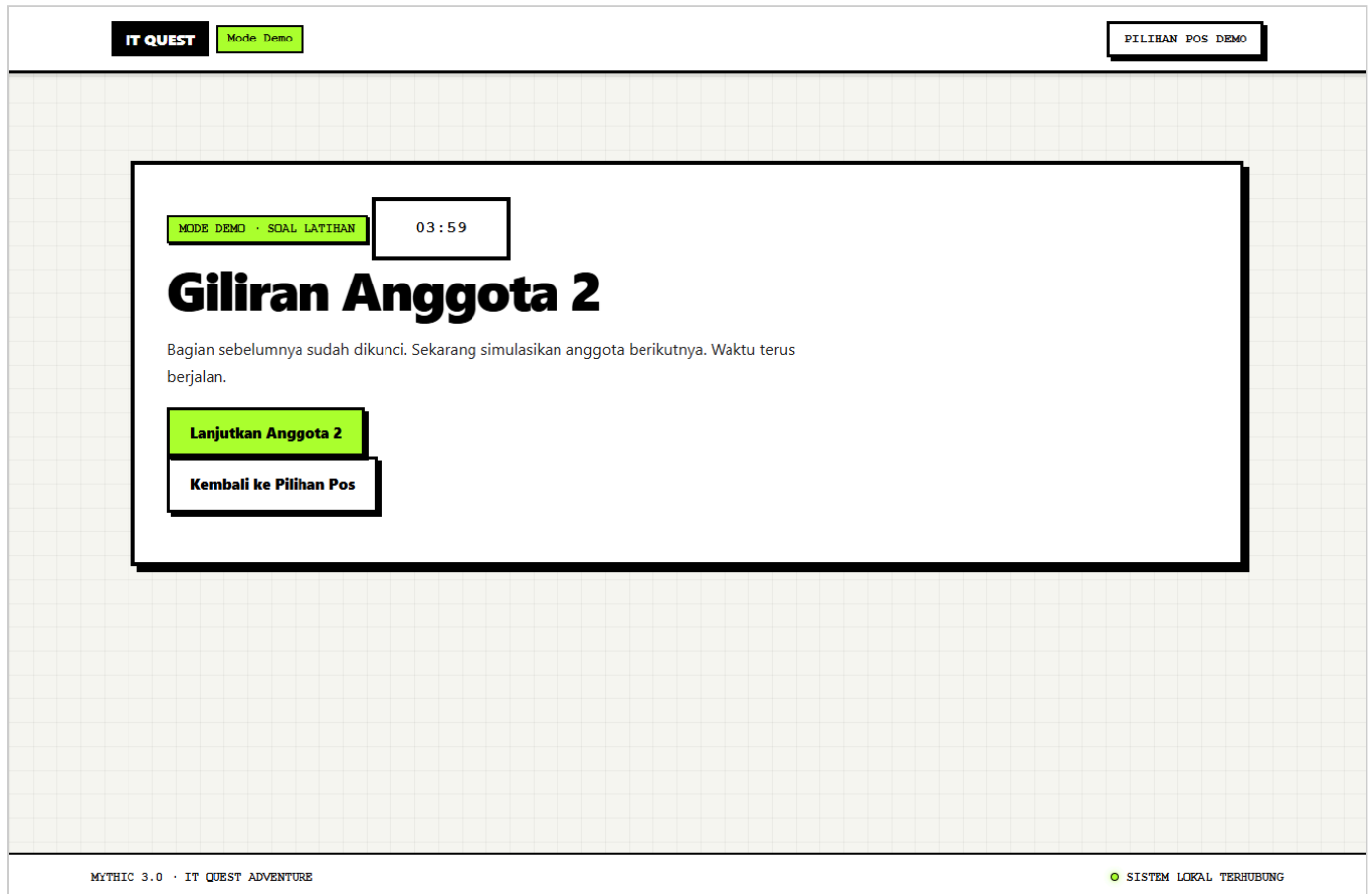
Gambar 6. Halaman pergantian menuju Anggota 2; alur yang sama digunakan menuju Anggota 3.
