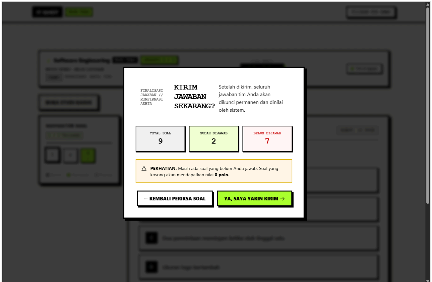
Gambar 7. Dialog konfirmasi submit; soal yang masih kosong mendapat 0 poin.
