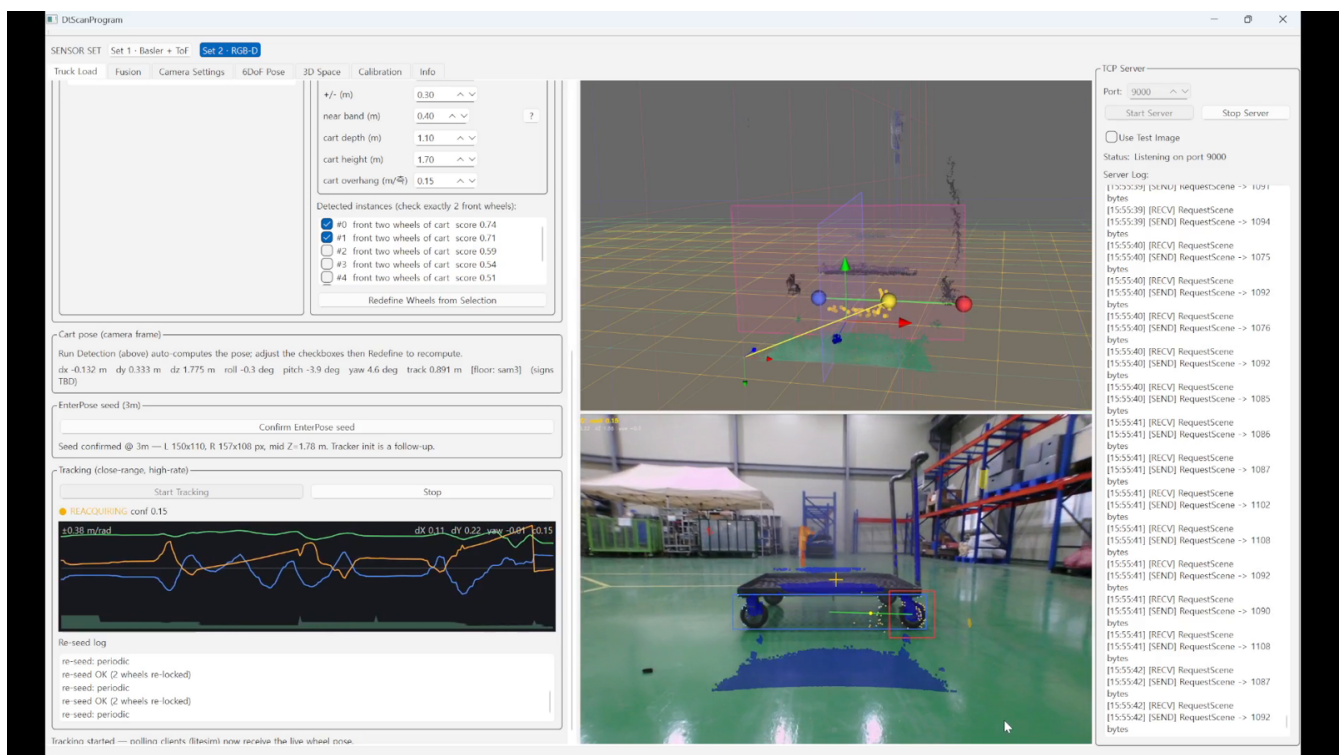
그림 1. 무인지게차 DOTORI의 비전 서버링 테스트 화면 녹화입니다(3D 뷰-카메라 영상-신호 플롯).
