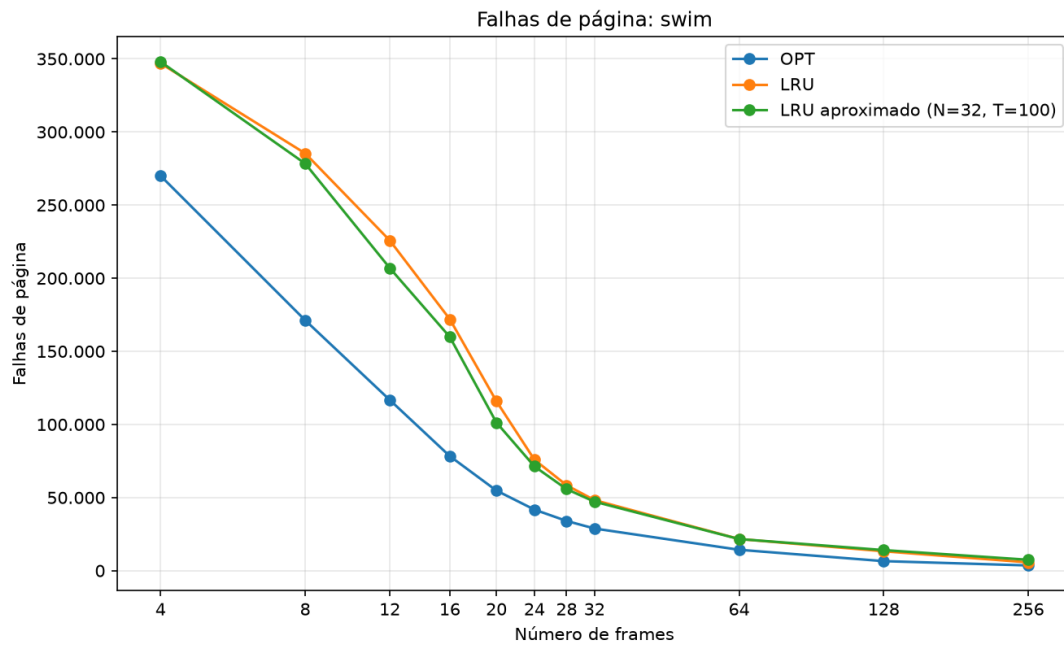
Figura 5: falhas de página no trace swim.
