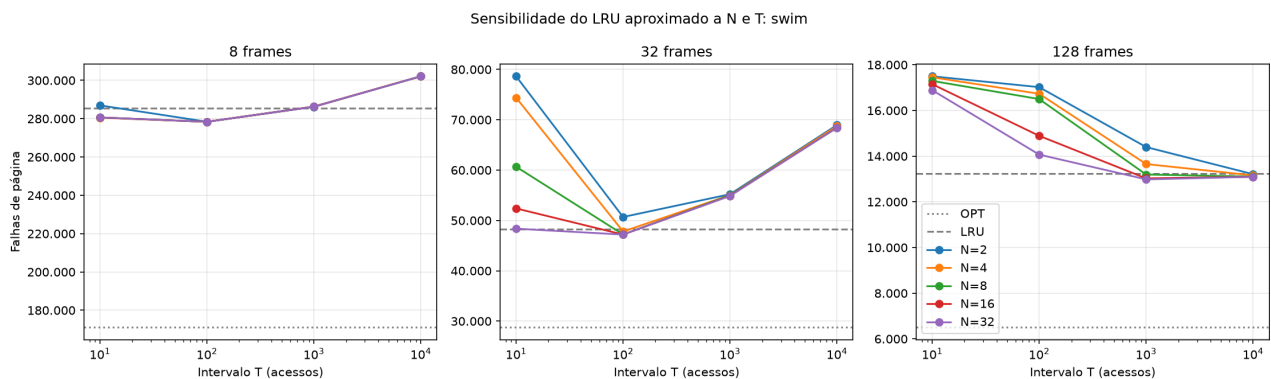
Figura 1: falhas do LRU aproximado em função de T no trace swim. As linhas tracejada e pontilhada indicam o LRU exato e o OPT.
