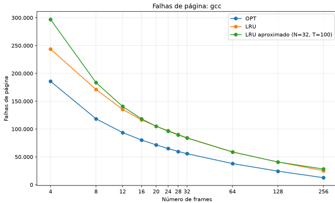
Figura 3: falhas de página no trace gcc.
