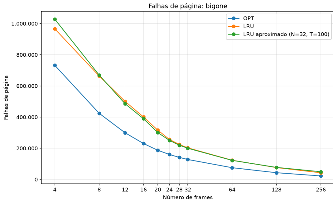
Figura 6: falhas de página no trace bigone.
