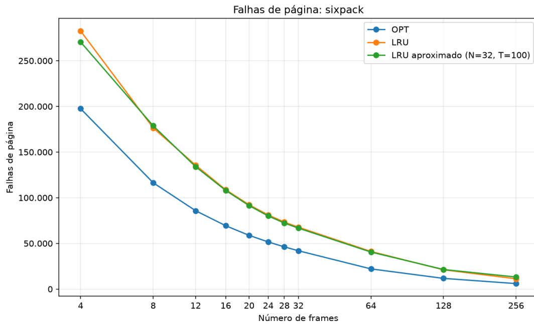
Figura 4: falhas de página no trace sixpack.
