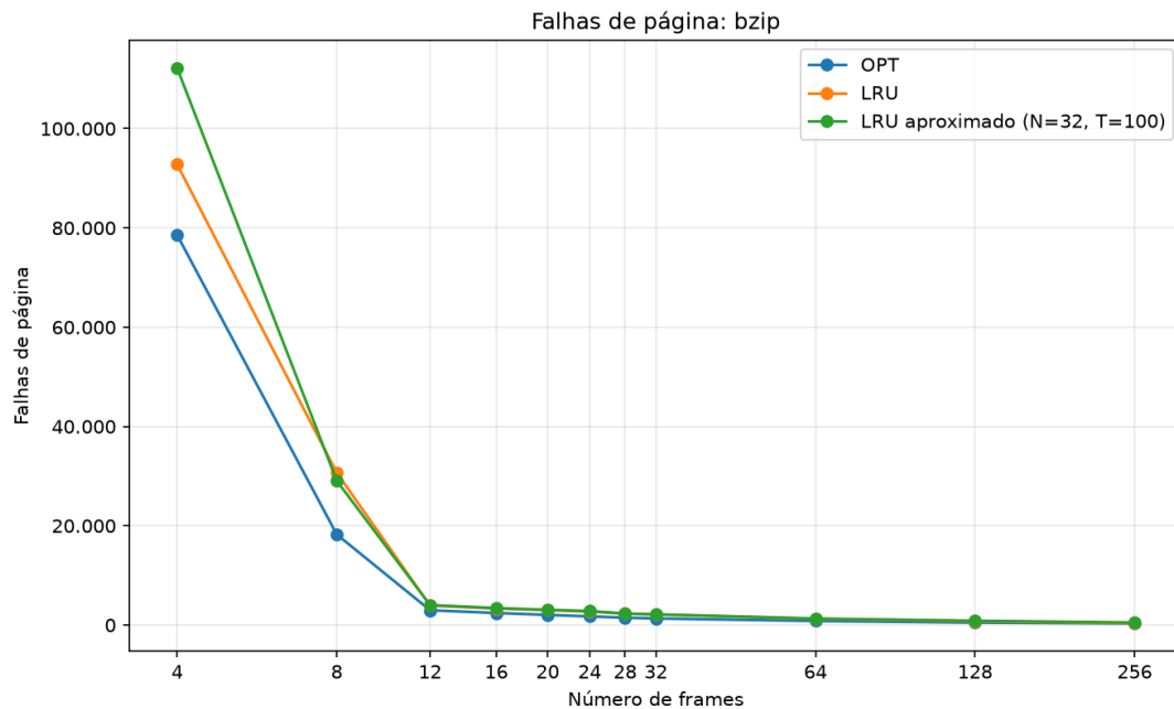
Figura 2: falhas de página no trace bzip.
