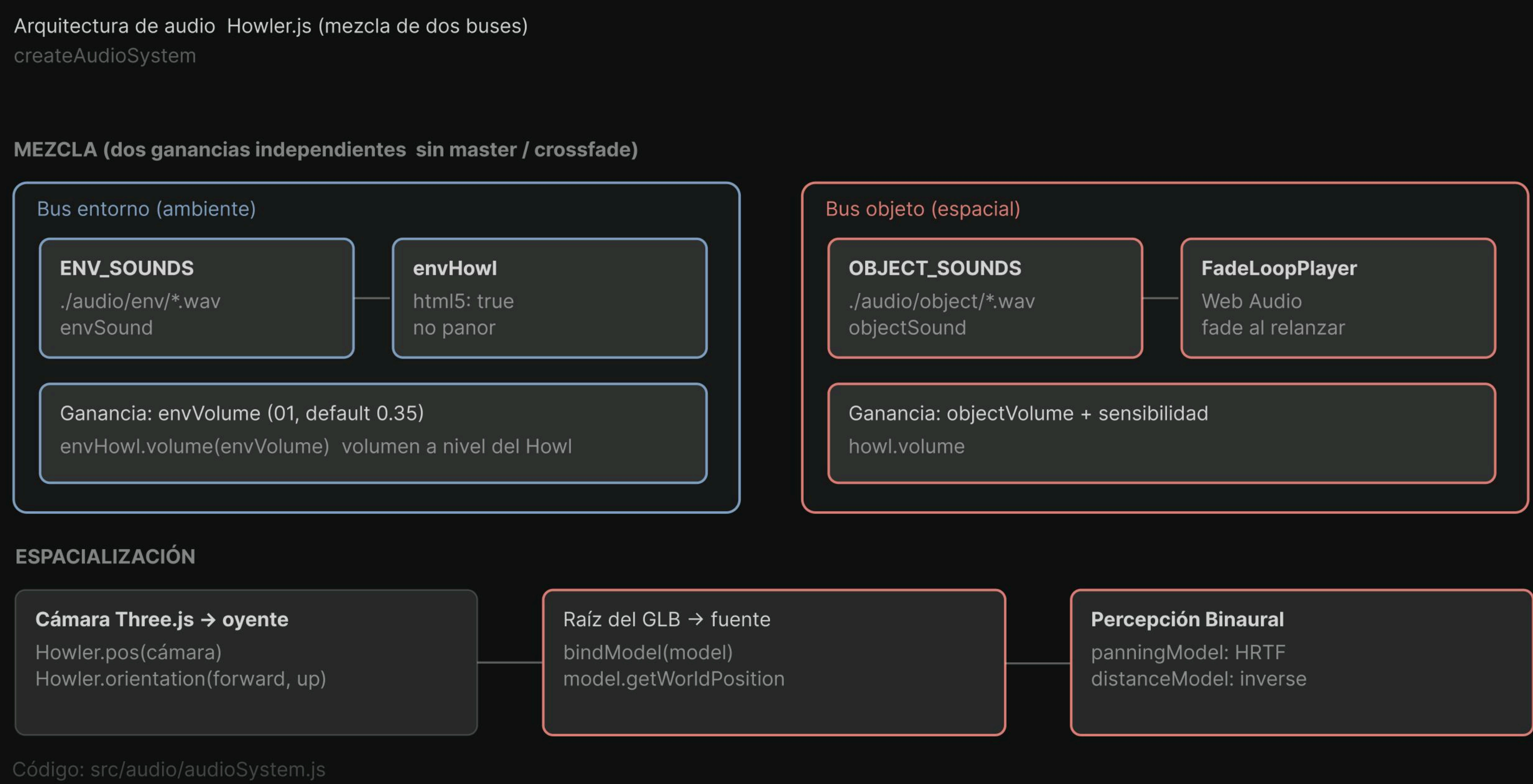
fig 12: Diagrama de implementación de arquitectura de audio usando Howler.js
