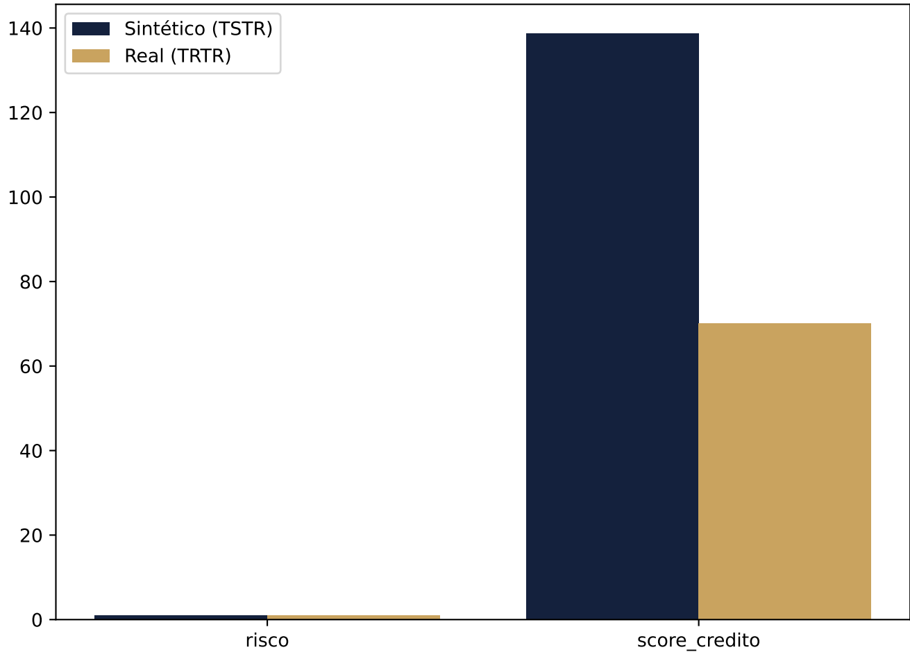
Utilidade por tarefa: Sintético vs. Real
