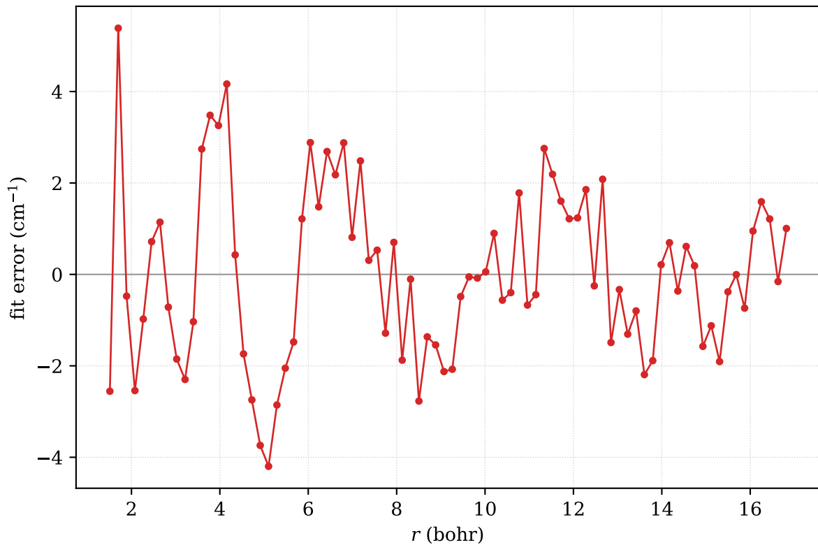
Rydberg-6 fit error (fit - ab initio), RMS = 1.86 cm -1
