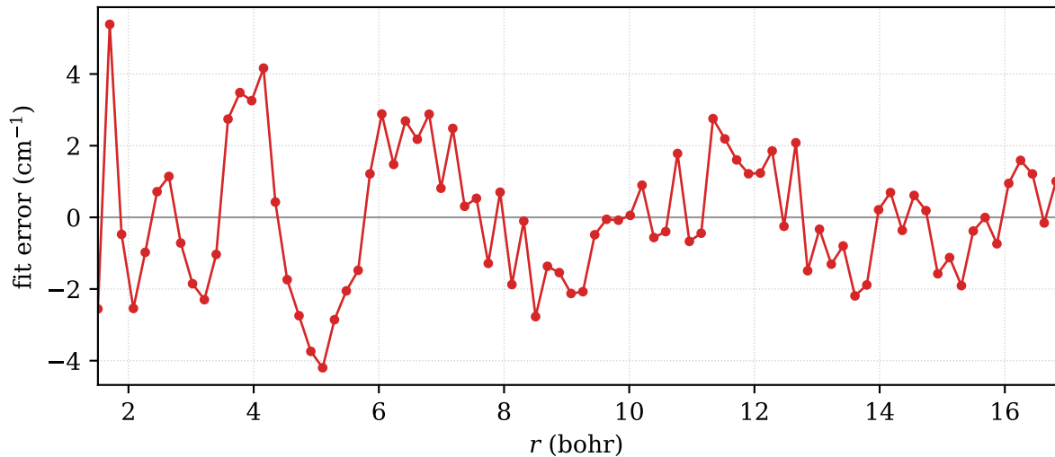
Rydberg-6 fit error (fit – ab initio), RMS = 1.86 cm -1
