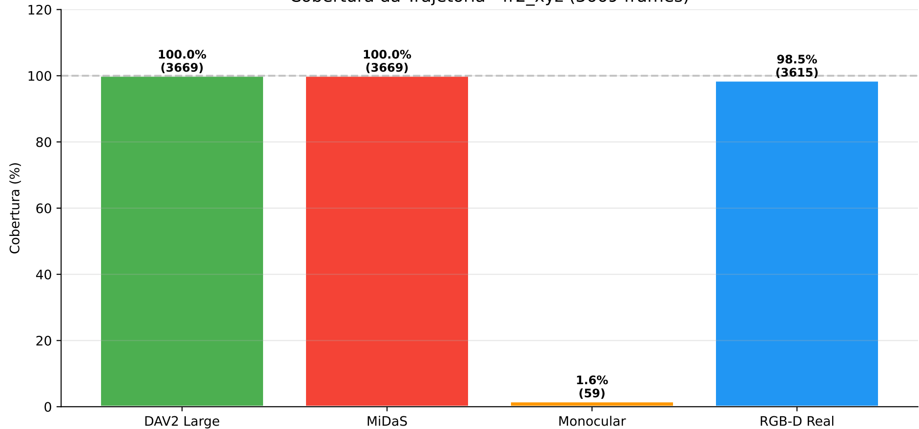
Cobertura da Trajetoria - fr2_xyz (3669 frames)
