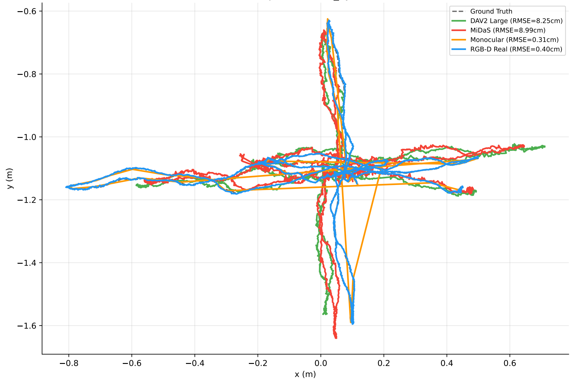
Trajetorias - fr2_xyz
