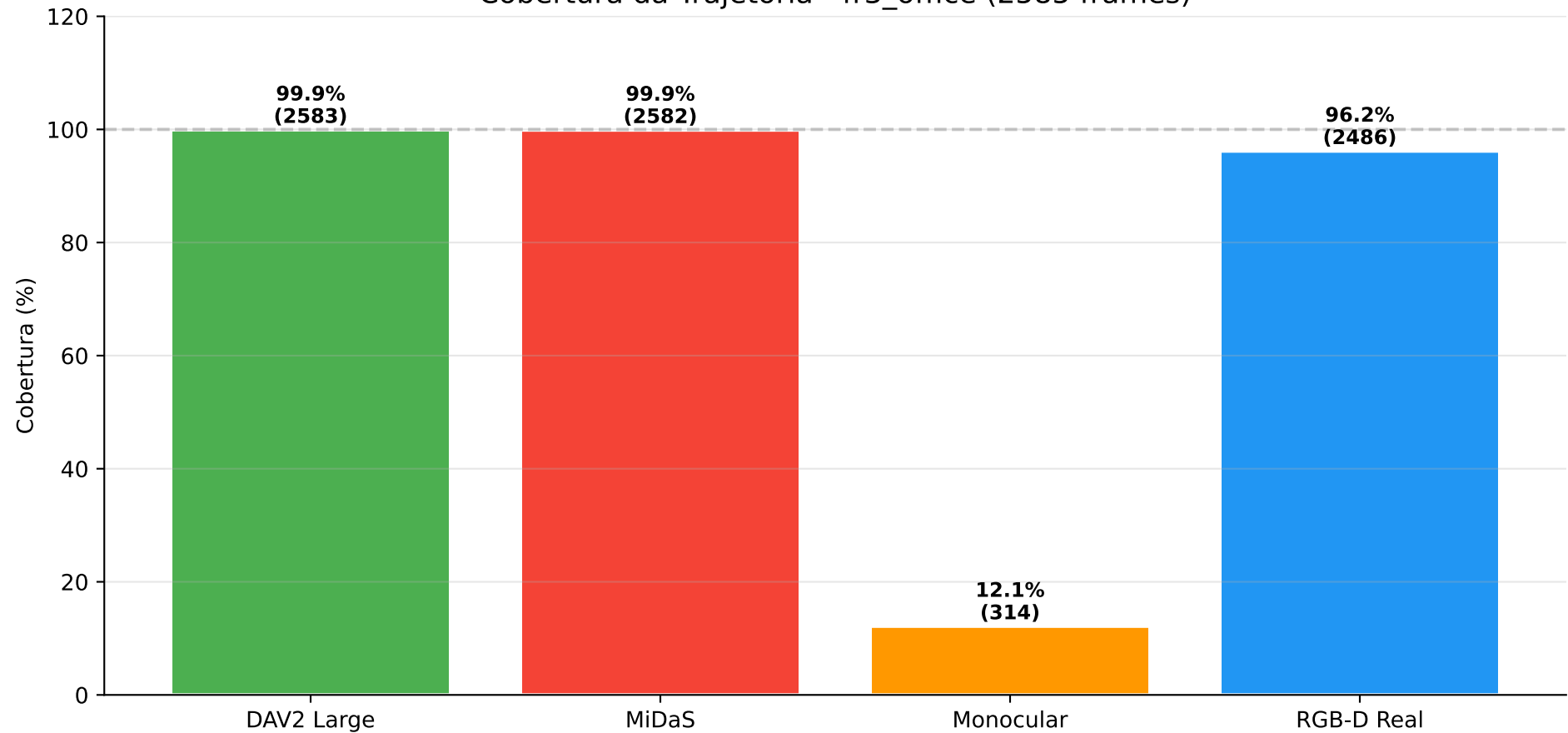
Cobertura da Trajetoria - fr3_office (2585 frames)
