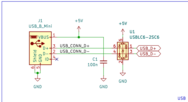
USB
