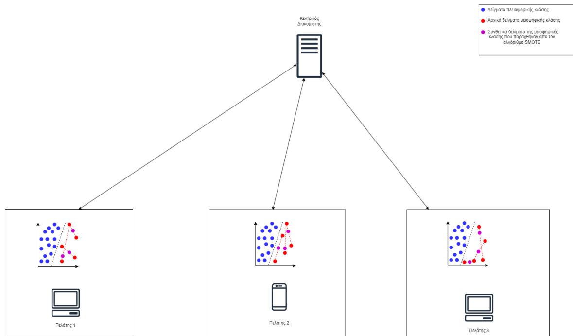
Σχήμα 3.6: Αναπαράσταση Προσέγγισης Client-Side SMOTE
