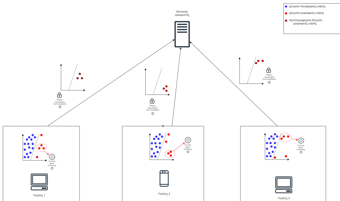
Σχήμα 3.7: Αναπαράσταση Προσέγγισης Trans-Client SMOTE - Μέρος 1ο
