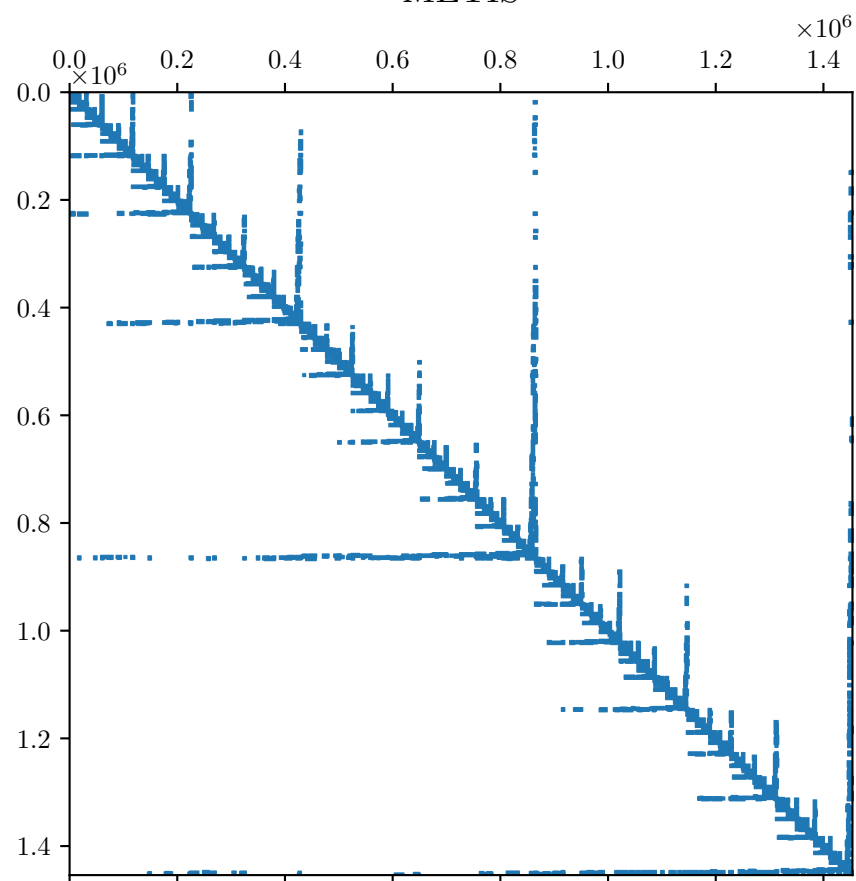
METIS
