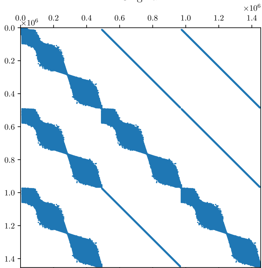
AMD
