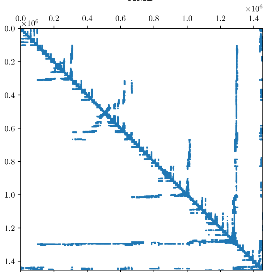
AMD
