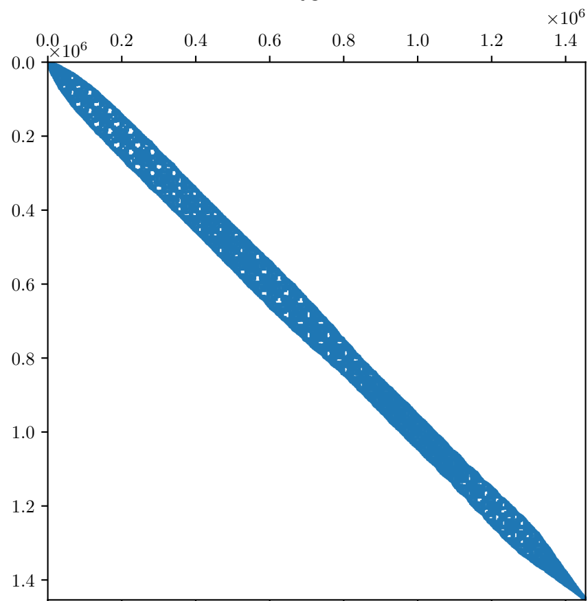
METIS
