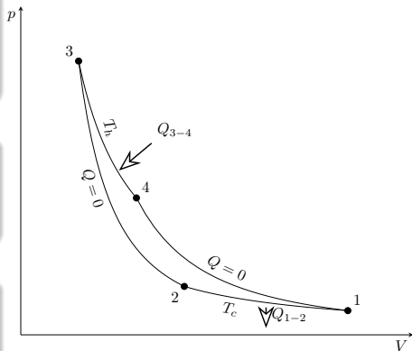
Schemat silnika Carnota 1
