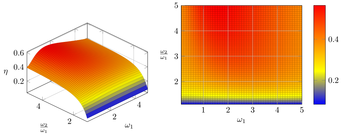
Rys. 2.6. Wykres sprawności kwantowego silnika Stirlinga z układem o spinie \frac{1}{2} jako czynnika roboczym i bez regeneratora; wykorzystano jednostki naturalne k_B = 1 , \hbar = 1 ; stosunek temperatur jest równy \frac{T_h}{T_c} = 3 ; dla silnika Carnota \eta_C = \frac{2}{3} .
