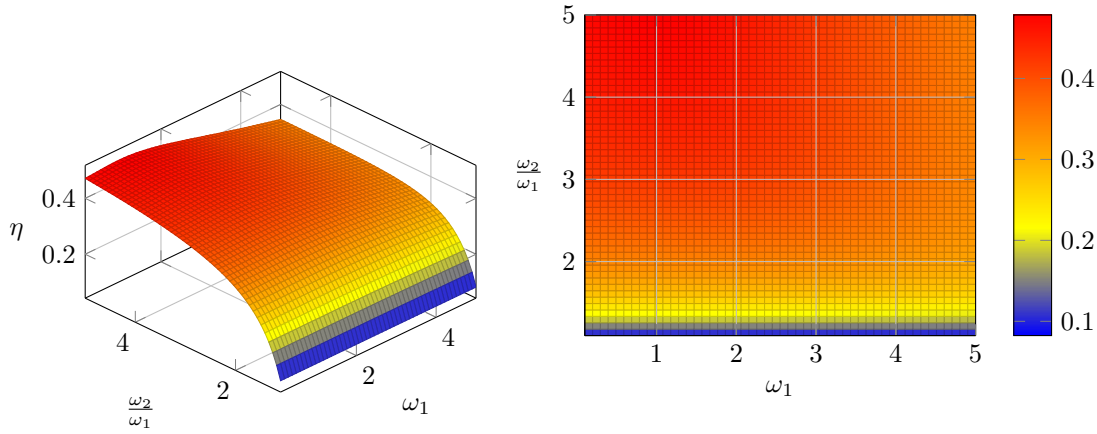
Rys. 2.4. Wykres sprawności kwantowego silnika Stirlinga z oscylatorem harmonicznym jako czynnikiem roboczym i bez regeneratora; wykorzystano jednostki naturalne k_B = 1 , \hbar = 1 ; stosunek temperatur jest równy \frac{T_h}{T_c} = 3 ; dla silnika Carnota \eta_C = \frac{2}{3} .
