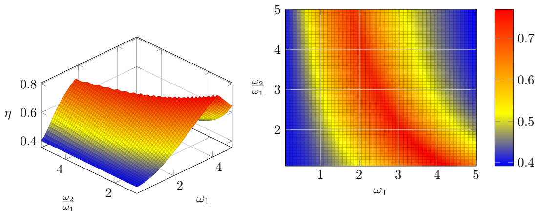
Rys. 2.5. Wykres sprawności kwantowego silnika Stirlinga z układem o spinie \frac{1}{2} jako czynnika roboczym; wykorzystano jednostki naturalne k_B = 1 , \hbar = 1 ; stosunek temperatur jest równy \frac{T_h}{T_c} = 3 ; dla silnika Carnota \eta_C = \frac{2}{3} .
