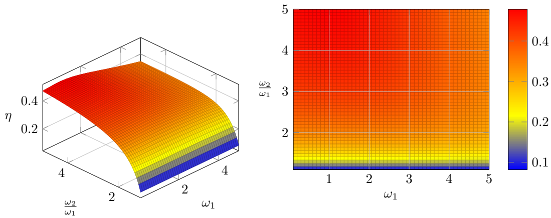
Rys. 2.4. Wykres sprawności kwantowego silnika Stirlinga z oscylatorem harmonicznym jako czynnikiem roboczym i bez regeneratora; wykorzystano jednostki naturalne k_B = 1 , \hbar = 1 ; stosunek temperatur jest równy \frac{T_h}{T_c} = 3 .
