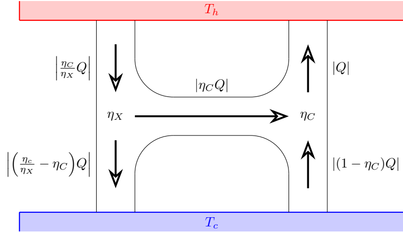
Rys. 1.6. Schemat podwójnego silnika
