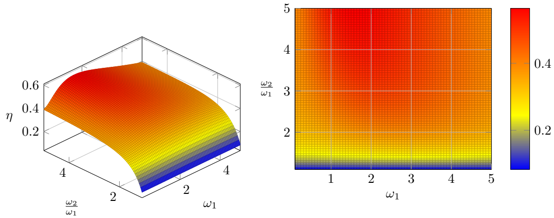
Rys. 2.7. Wykres sprawności kwantowego silnika Stirlinga z układem o spinie \frac{1}{2} jako czynnikiem roboczym i bez regeneratora; wykorzystano jednostki naturalne k_B = 1 , \hbar = 1 ; stosunek temperatur jest równy \frac{T_h}{T_c} = 3 ; w tych warunkach sprawność silnika Carnota jest równa \eta_C = \frac{2}{3} .
