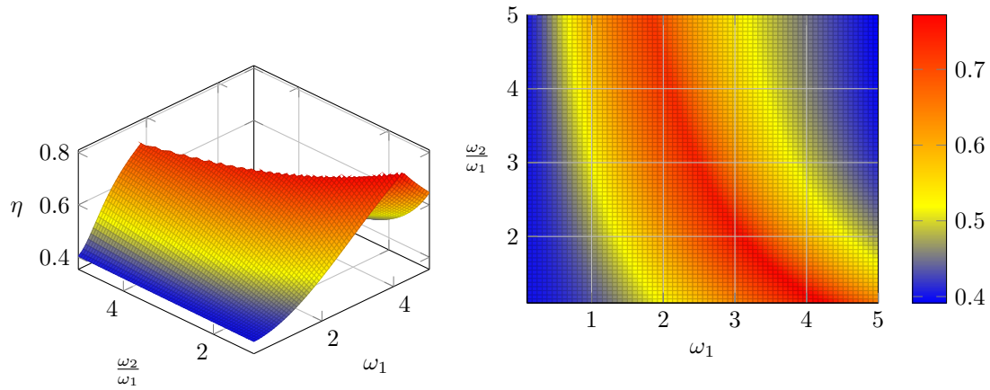
Rys. 2.6. Wykres sprawności kwantowego silnika Stirlinga z układem o spinie \frac{1}{2} jako czynnikiem roboczym; wykorzystano jednostki naturalne k_B = 1 , \hbar = 1 ; stosunek temperatur jest równy \frac{T_h}{T_c} = 3 ; w tych warunkach sprawność silnika Carnota jest równa \eta_C = \frac{2}{3} .
