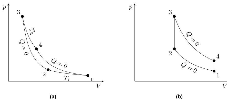
Rys. 1.2. Porównanie wykresów cykli prawobieżnych: (a) Carnota i (b) Otto.
