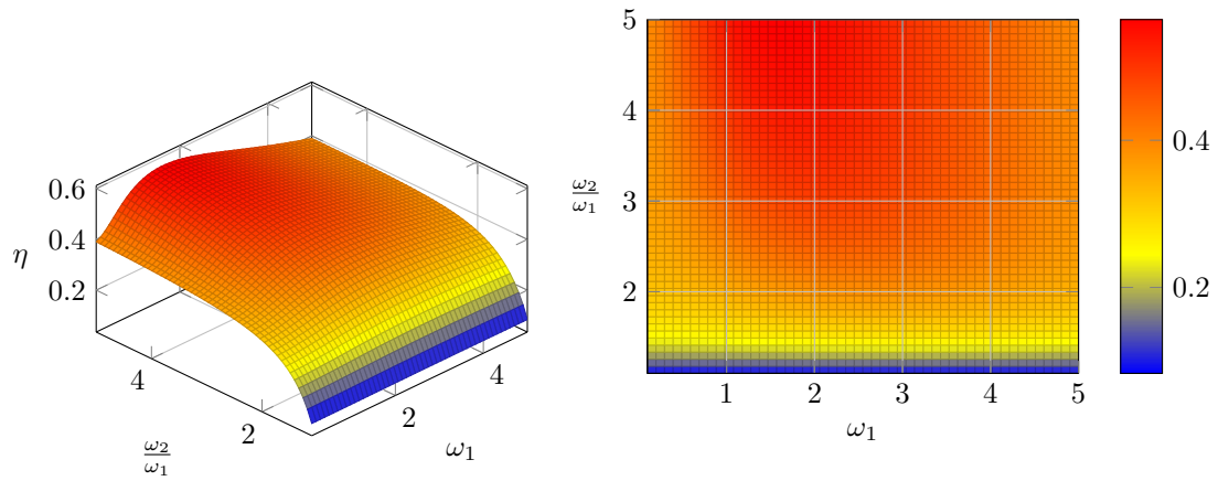
Rys. 2.6. Wykres sprawności kwantowego silnika Stirlinga z układem o spinie \frac{1}{2} jako czynnika roboczym i bez regeneratora; wykorzystano jednostki naturalne k_B = 1 , \hbar = 1 ; stosunek temperatur jest równy \frac{T_h}{T_c} = 3 ; dla silnika Carnota \eta_C = \frac{2}{3} .
