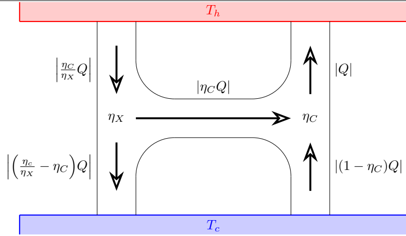
Rys. 1.3. Schemat podwójnego silnika
