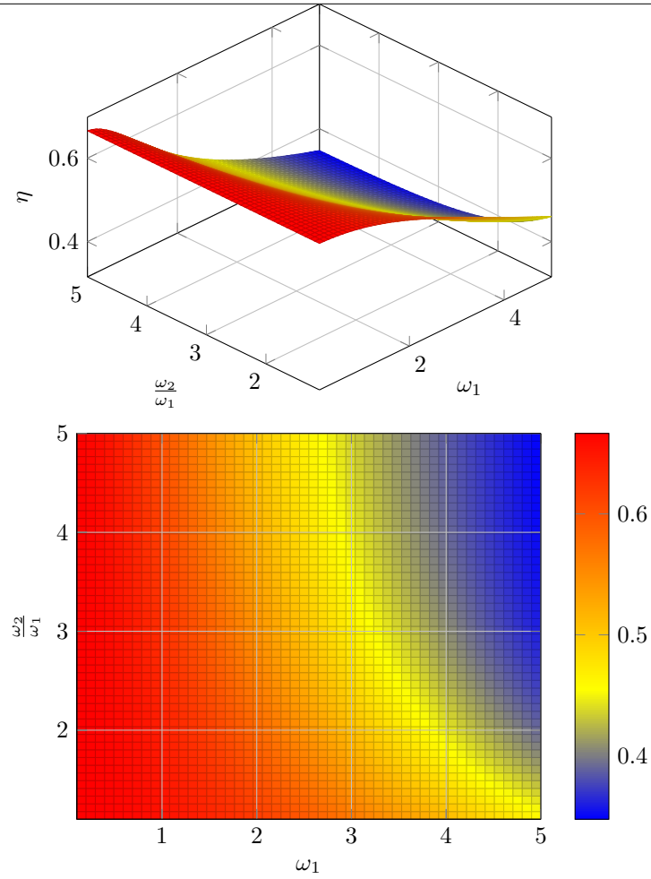
Rys. 2.3. Wykres sprawności kwantowego silnika Stirlinga z oscylatorem harmonicznym jako czynnikiem roboczym
