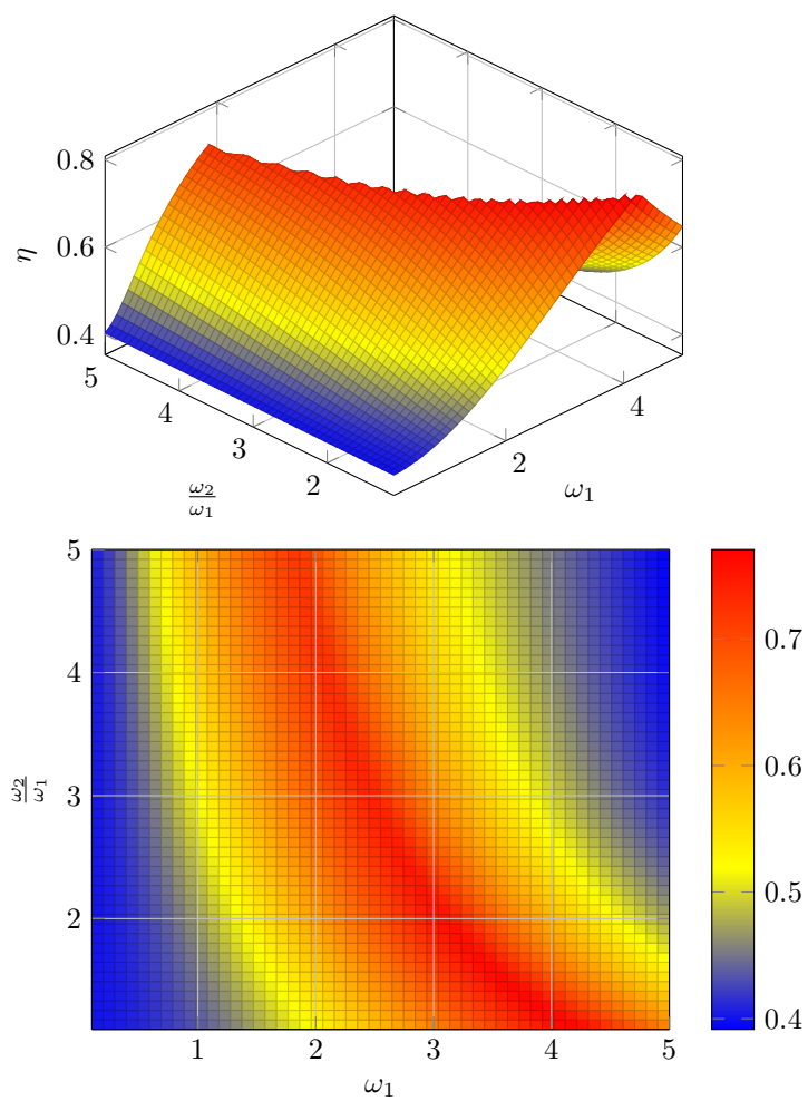
Rys. 2.4. Wykres sprawności kwantowego silnika Stirlinga z układem o spinie \frac{1}{2} jako czynnika roboczym
