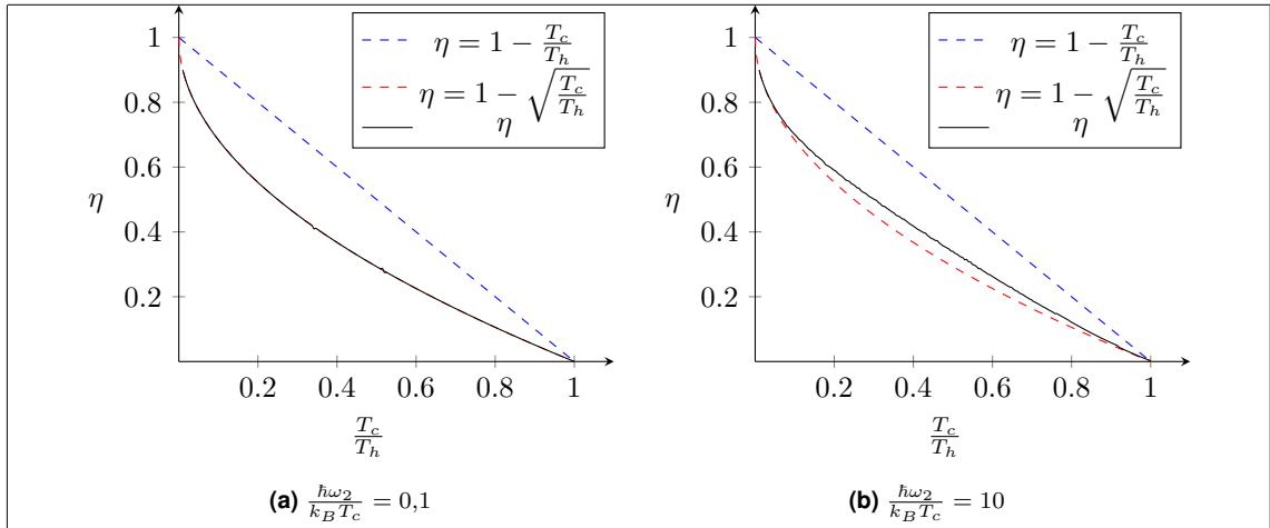
Rys. 2.1. Porównanie sprawności silnika Otto w przypadku wysokotemperaturowym (a) oraz niskotemperaturowym (b).
