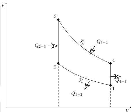
Schemat silnika Stirlinga
