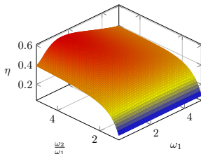
Rysunek: Silnik Stirlinga ze spinem \frac{1}{2}
