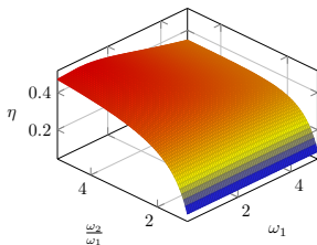
Rysunek: Silnik Stirlinga z oscylatorem harmonicznym
