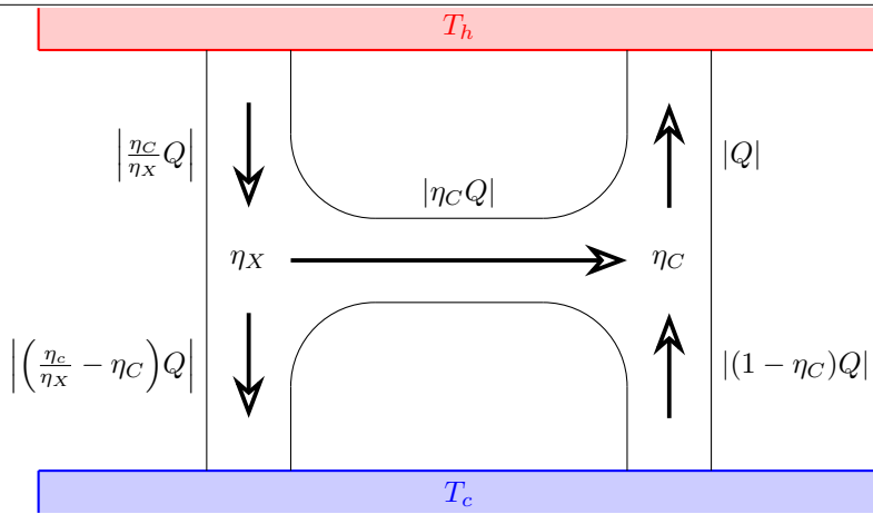
Rys. 1.3. Schemat podwójnego silnika
