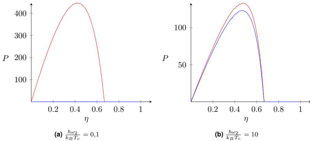
Rys. 2.3. Porównanie mocy silnika Otto w przypadku wysokotemperaturowym (a) oraz niskotemperaturowym (b).
