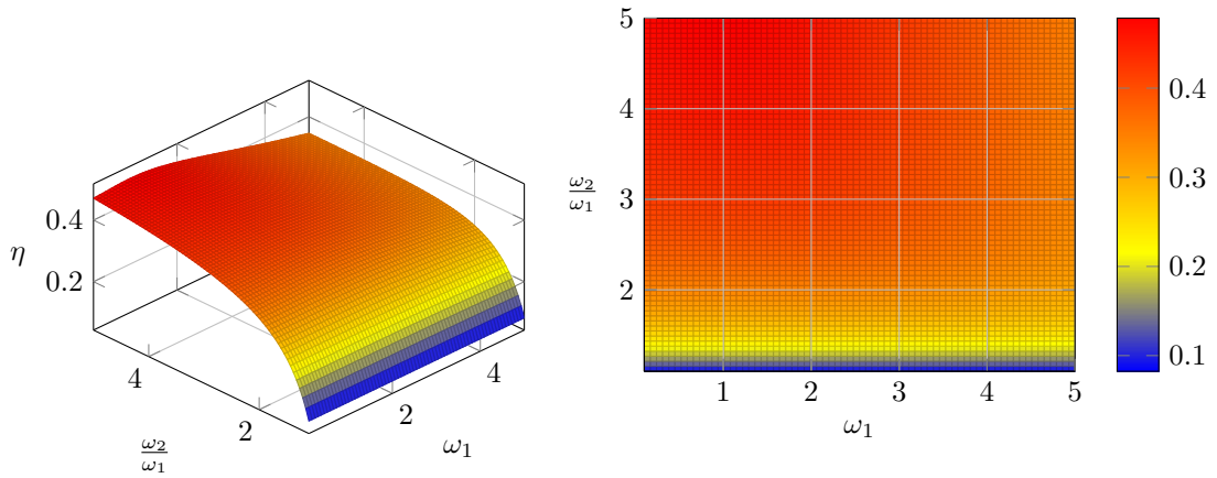
Rys. 3.5. Wykres sprawności kwantowego silnika Stirlinga z oscylatorem harmonicznym jako czynnikiem roboczym i bez regeneratora; wykorzystano jednostki naturalne k_B = 1 , \hbar = 1 ; stosunek temperatur jest równy \frac{T_h}{T_c} = 3 ; w tych warunkach sprawność silnika Carnota jest równa \eta_C = \frac{2}{3} .
