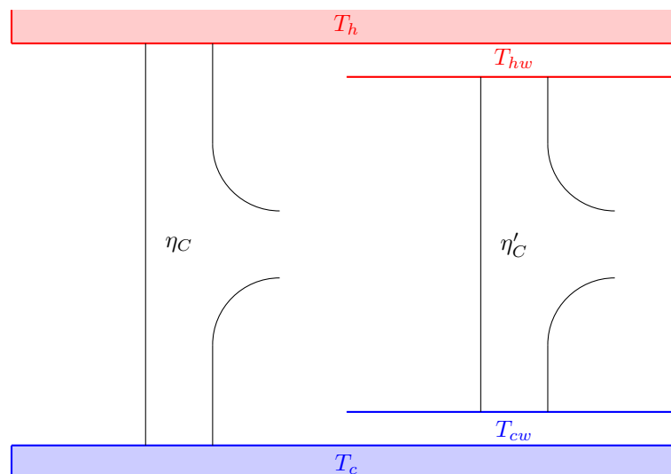
Rys. 2.7. Schemat porównawczy silnika Carnota odwracalnego (po lewej) oraz endoodwracalnego (po prawej).
