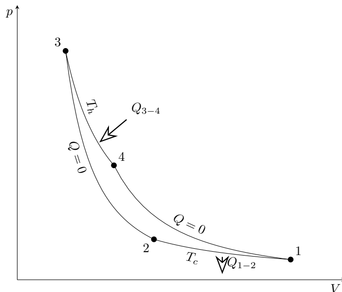
Rys. 2.3. Wykres cyklu Carnota w obiegu prawobieżnym.
