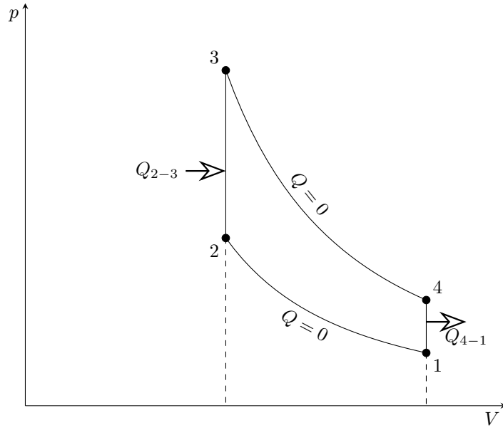
Rys. 2.4. Wykres cyklu Otto w obiegu prawobieżnym.
