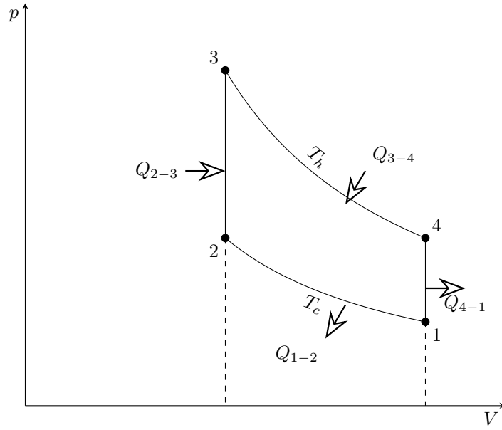
Rys. 2.5. Wykres cyklu Stirlinga w obiegu prawobieżnym.
