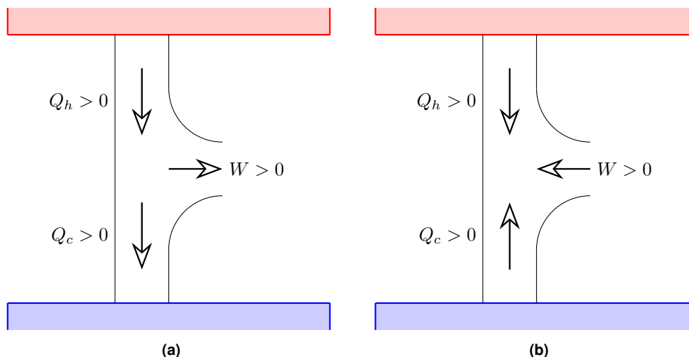
Rys. 2.2. Porównanie konwencji znaków: techniczna (a) i statystyczna (b).
