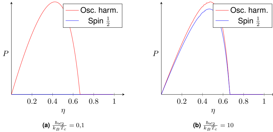
Rys. 3.3. Porównanie mocy silnika Otto w przypadku wysokotemperaturowym (a) oraz niskotemperaturowym (b).
