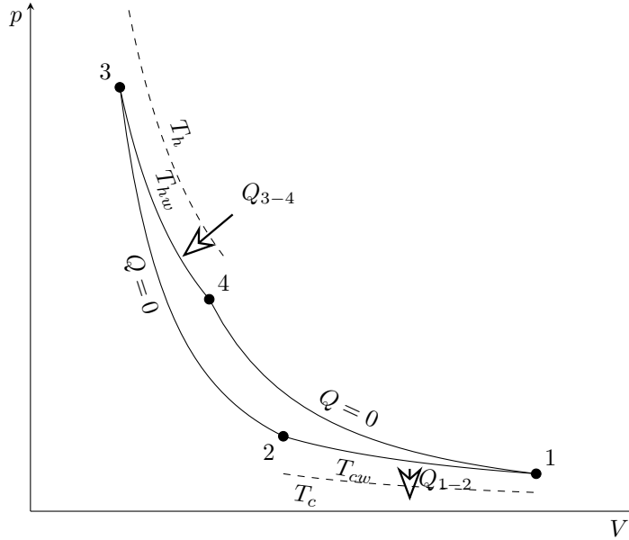
Rys. 2.8. Wykres cyklu Carnota w warunkach endoodwracalnych
