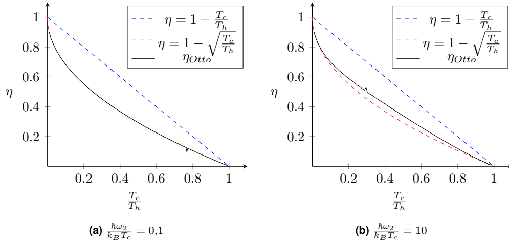
Rys. 3.1. Porównanie sprawności silnika Otto z oscylatorem harmonicznym jako czynnikiem roboczym w przypadku wysokotemperaturowym (a) oraz niskotemperaturowym (b).
