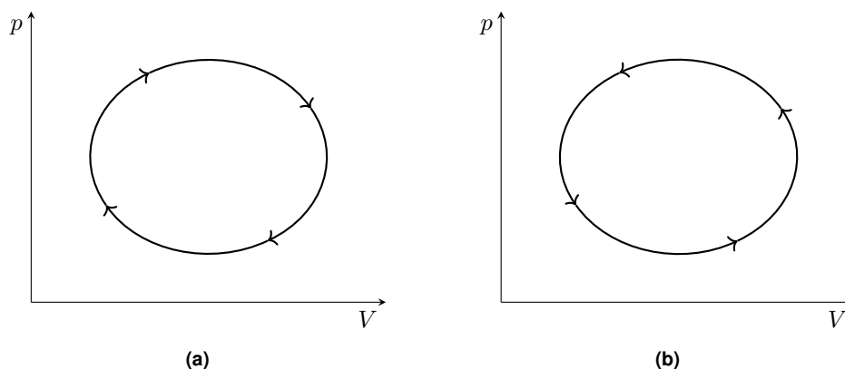
Rys. 2.1. Porównanie cyklu prawobieżnego (a) i lewobieżnego (b).
