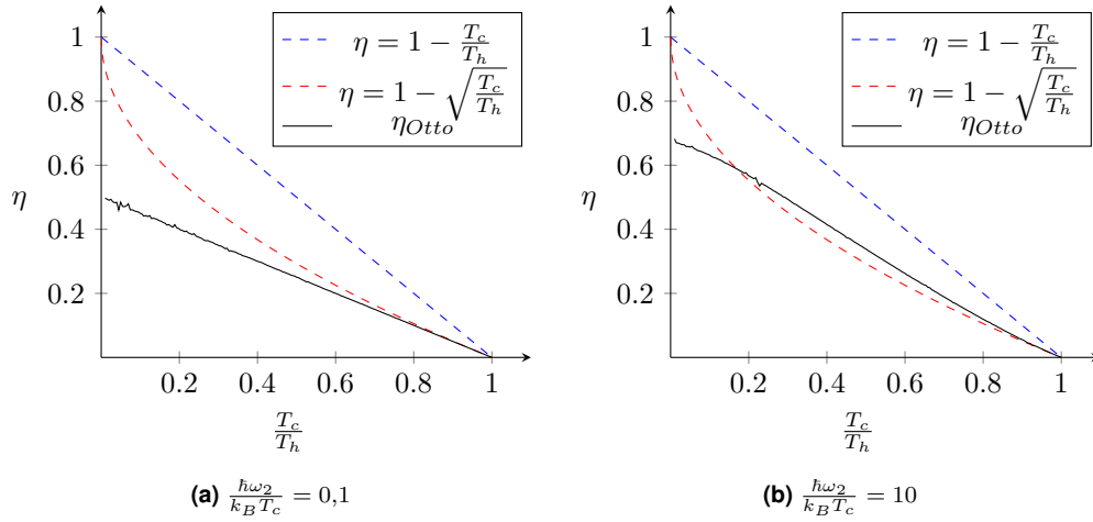
Rys. 3.2. Porównanie sprawności silnika Otto z układem o spinie \frac{1}{2} jako czynnikiem roboczym w przypadku wysokotemperaturowym (a) oraz niskotemperaturowym (b).
