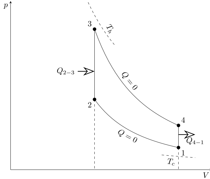
Rys. 2.9. Wykres cyklu Otto w warunkach endoodwracalnych
