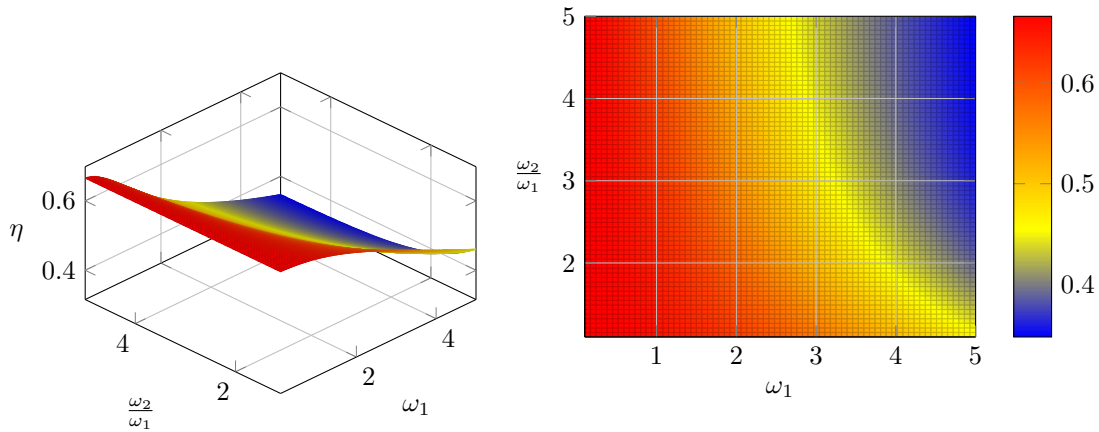
Rys. 3.4. Wykres sprawności kwantowego silnika Stirlinga z oscylatorem harmonicznym jako czynnikiem roboczym; wykorzystano jednostki naturalne k_B = 1 , \hbar = 1 ; stosunek temperatur jest równy \frac{T_h}{T_c} = 3 ; w tych warunkach sprawność silnika Carnota jest równa \eta_C = \frac{2}{3} .
