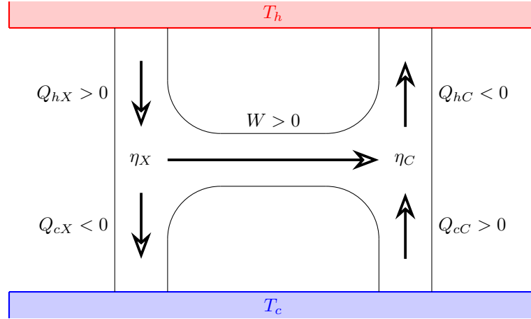
Rys. 2.6. Schemat podwójnego silnika
