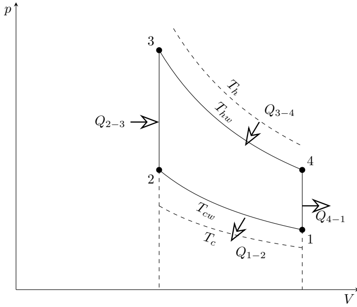
Rys. 2.10. Wykres cyklu Stirling w warunkach endoodwracalnych
