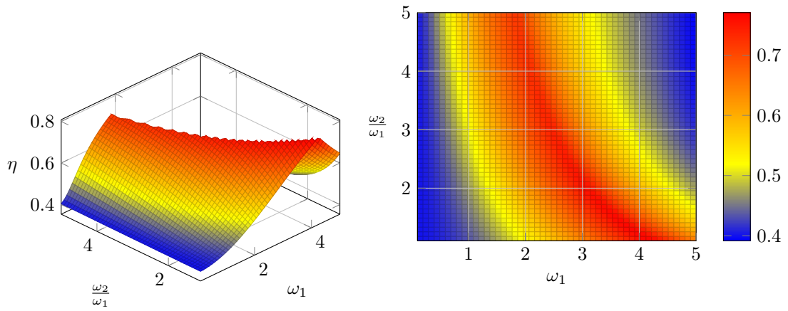
Rys. 2.4. Wykres sprawności kwantowego silnika Stirlinga z układem o spinie \frac{1}{2} jako czynnika roboczym; wykorzystano jednostki naturalne k_B = 1 , \hbar = 1 ; stosunek temperatur jest równy \frac{T_h}{T_c} = 3 .
