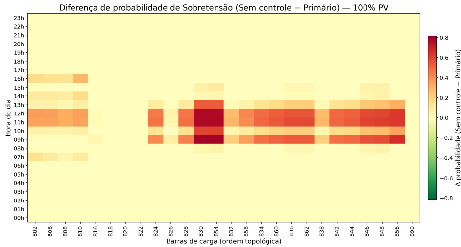
Figura 6.11: Diferença de probabilidade de sobretensão (sem controle — controle primário) por barra e hora, para 100% de penetração.
