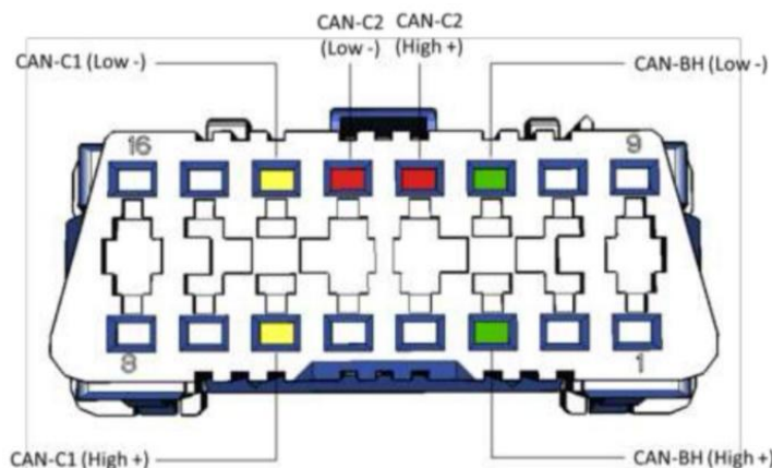
Connettore multiplo di Diagnosi DLC
