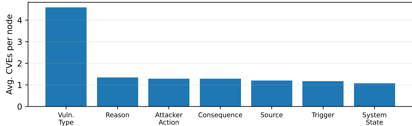
Semantic Reuse Distribution
