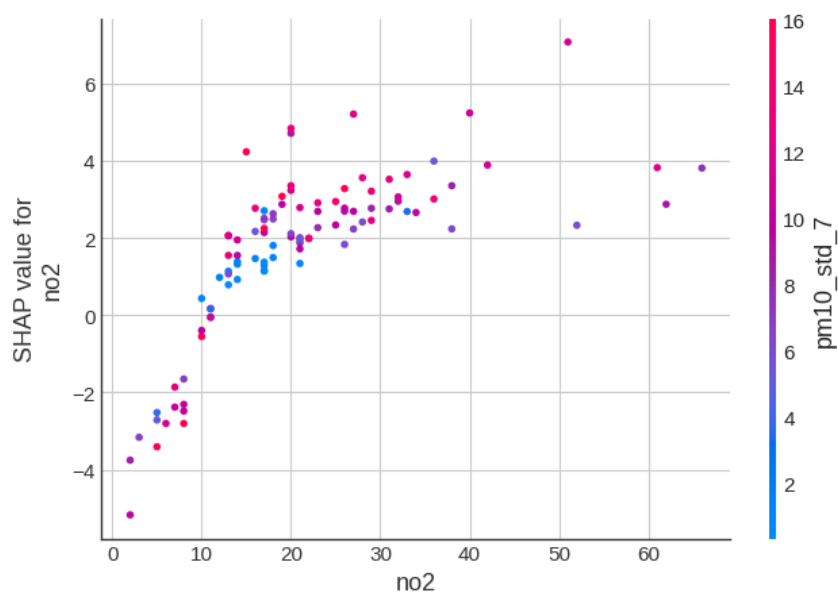
Gambar VI.10 SHAP Dependence Plot untuk Fitur Paling Berpengaruh
