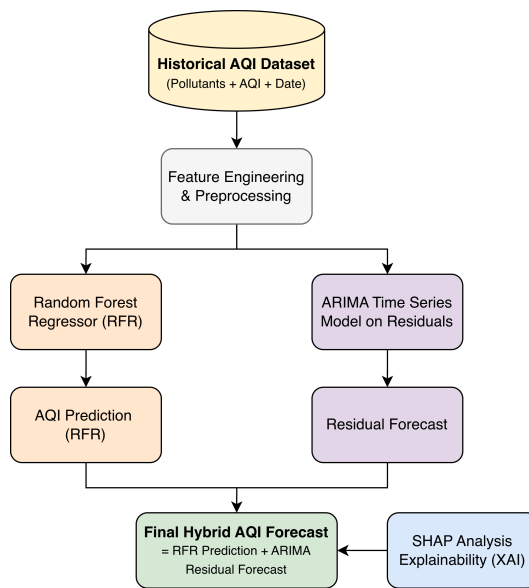
Gambar II.1 Arsitektur Aliran Kerja Model Hibrida Random Forest -ARIMA (Yenkikar dkk. Juli 2025)
