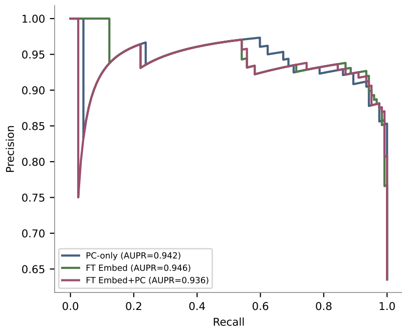
DILI
