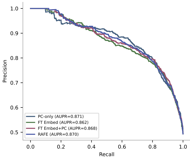
HERG
