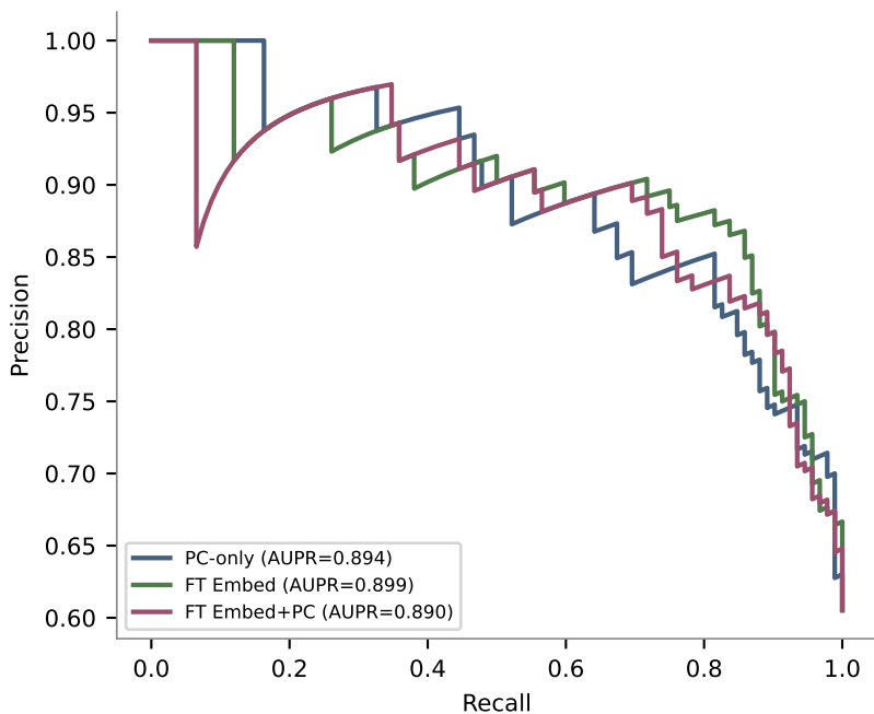
HERG
