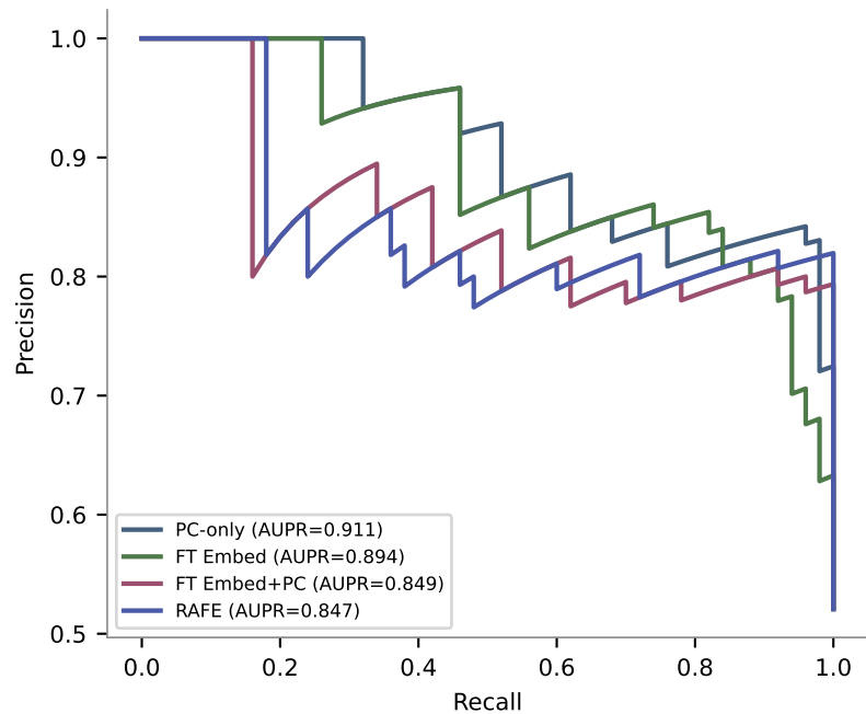
DILI
