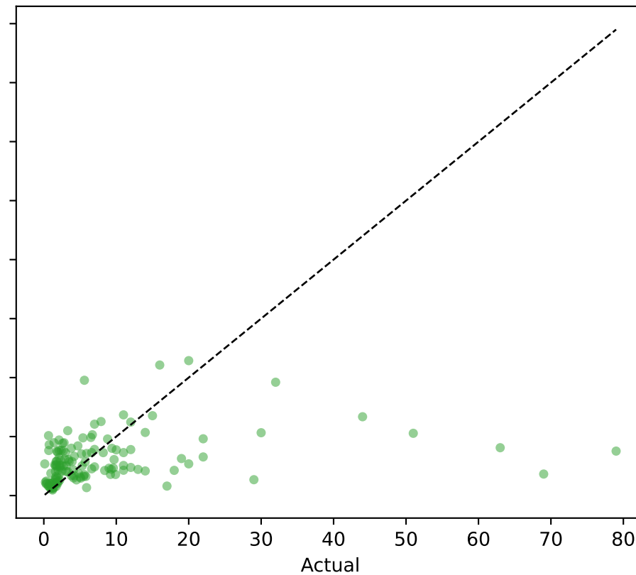
LightGBM (R2=0.065)
