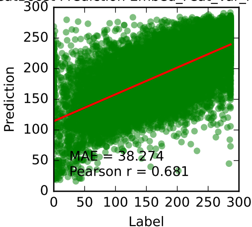
CatBoost Prediction Embed_Feat_Var_random
