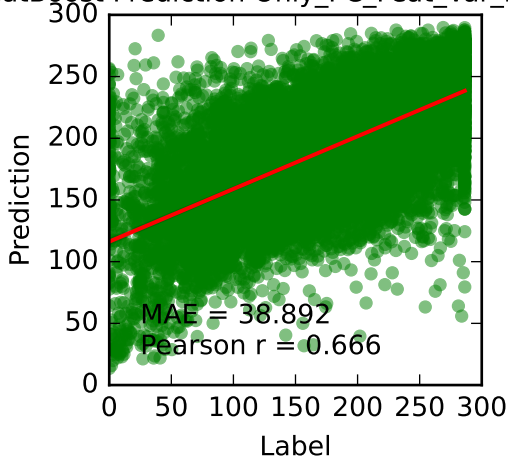
CatBoost Prediction Only_PC_Feat_Var_random
