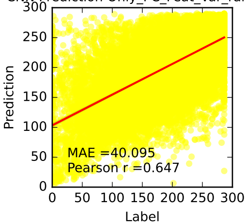
CNN Prediction Only_PC_Feat_Var_random
