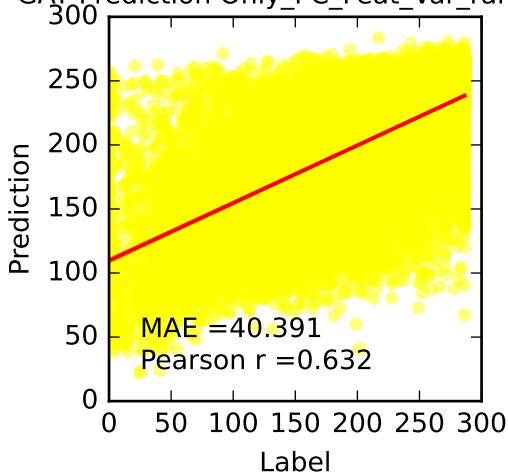
GAT Prediction Only_PC_Feat_Var_random
