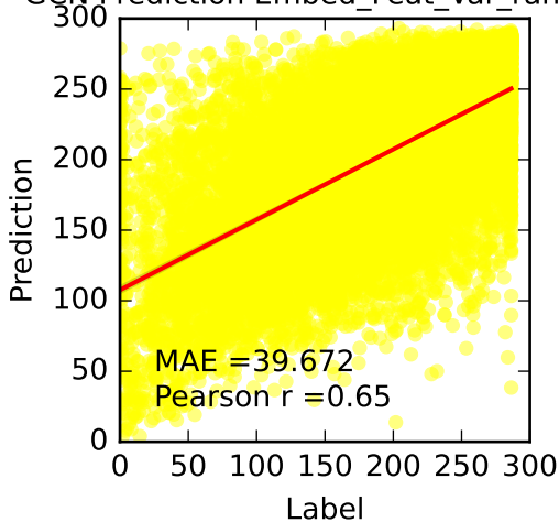
GCN Prediction Embed_Feat_Var_random
