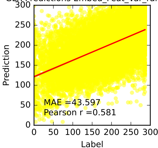
GLR Predictions Embed_Feat_Var_random
