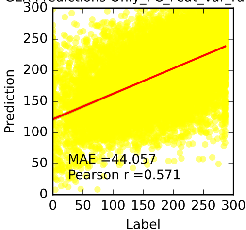
GLR Predictions Only_PC_Feat_Var_random
