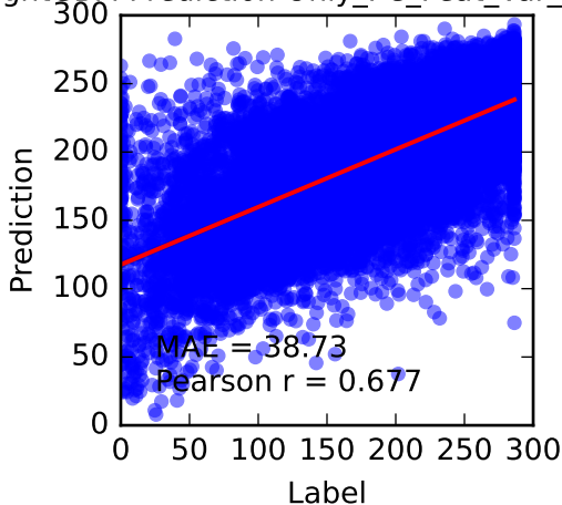
LightGBM Prediction Only_PC_Feat_Var_random
