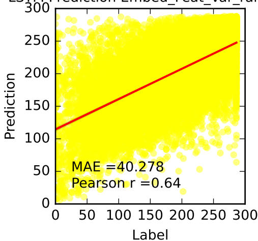
LSTM Prediction Embed_Feat_Var_random
