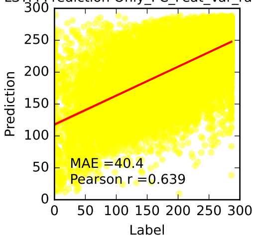
LSTM Prediction Only_PC_Feat_Var_random
