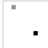
ch4 value
