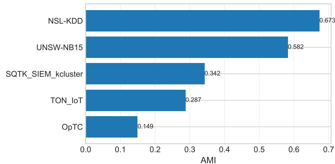
AMI
