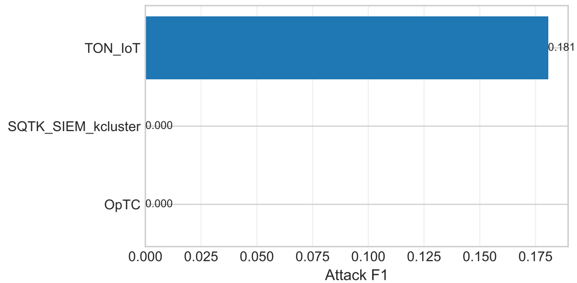
Attack F1
