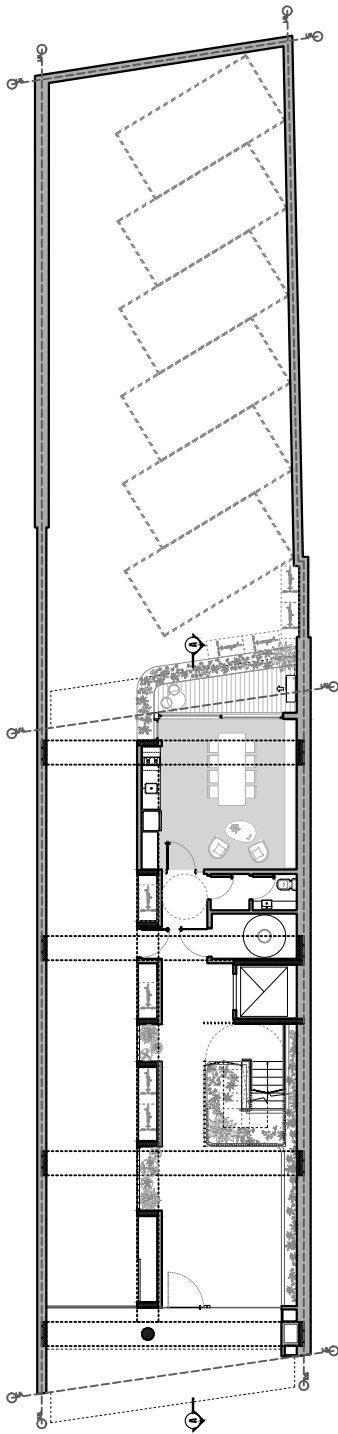
PLANTA BAJA
