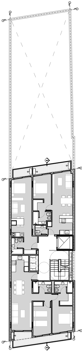
PLANTA TIPO (1°-4°)
