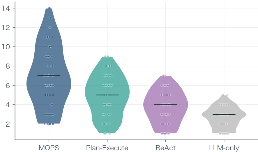
LLM 调用次数
